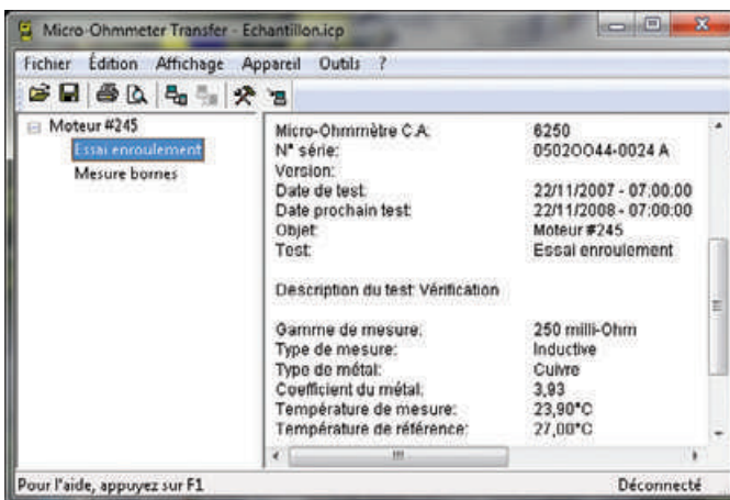
MODULE MOT Résultats sur test enroulement moteur
