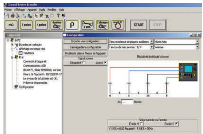
MODULE GTT Exemple de configuration
